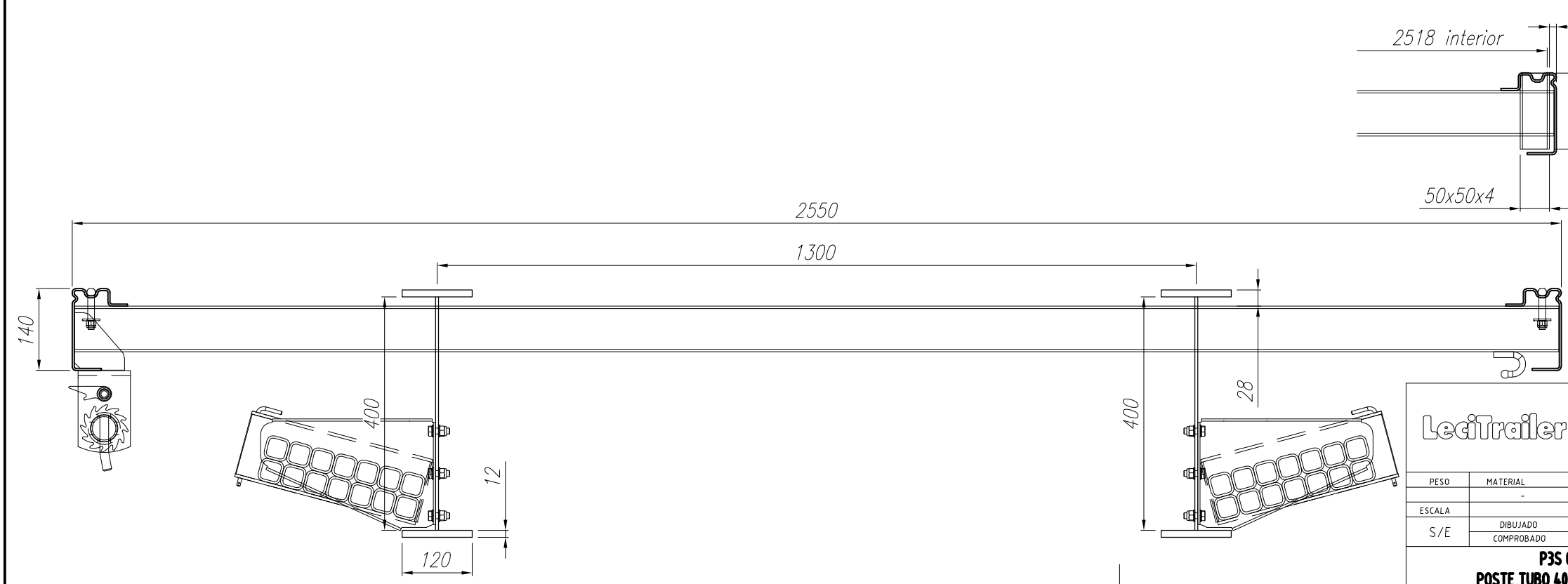
DETALLE CASQUILLO PARA POSTE TUBO 40x40
