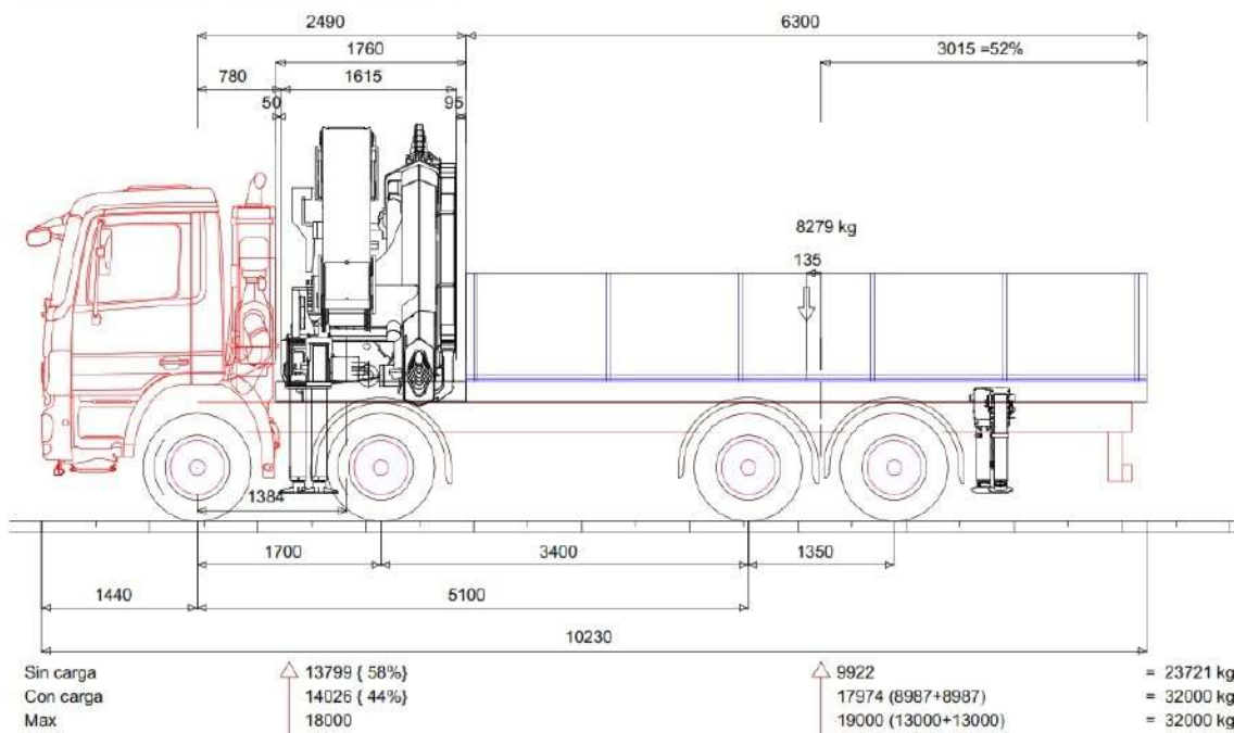
Mercedes-Benz S2 4141K 8X4/4
